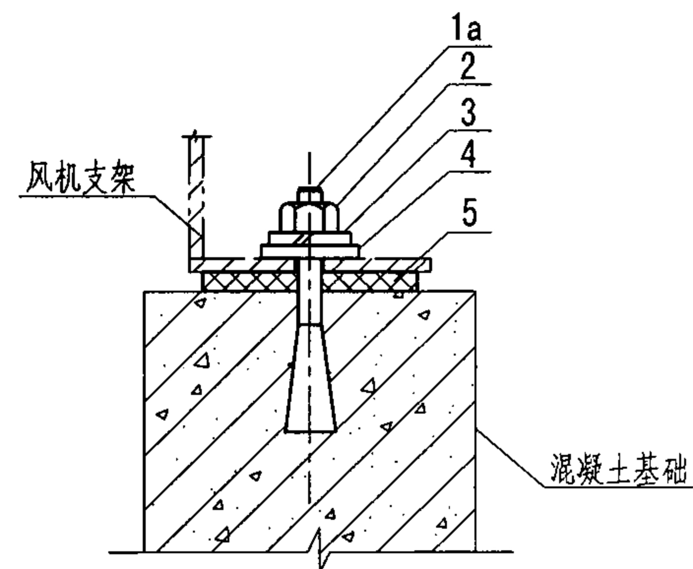
① 胀锚螺栓安装
