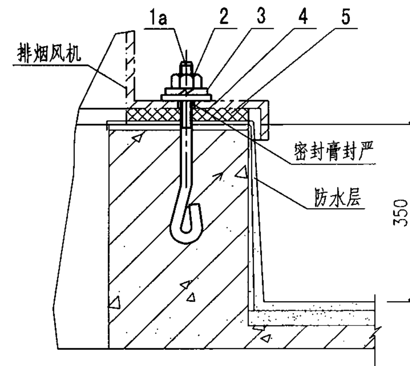
① 地脚螺栓安装
