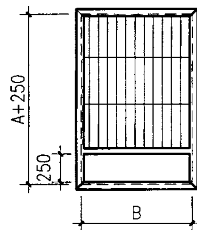
排烟口垂直安装
