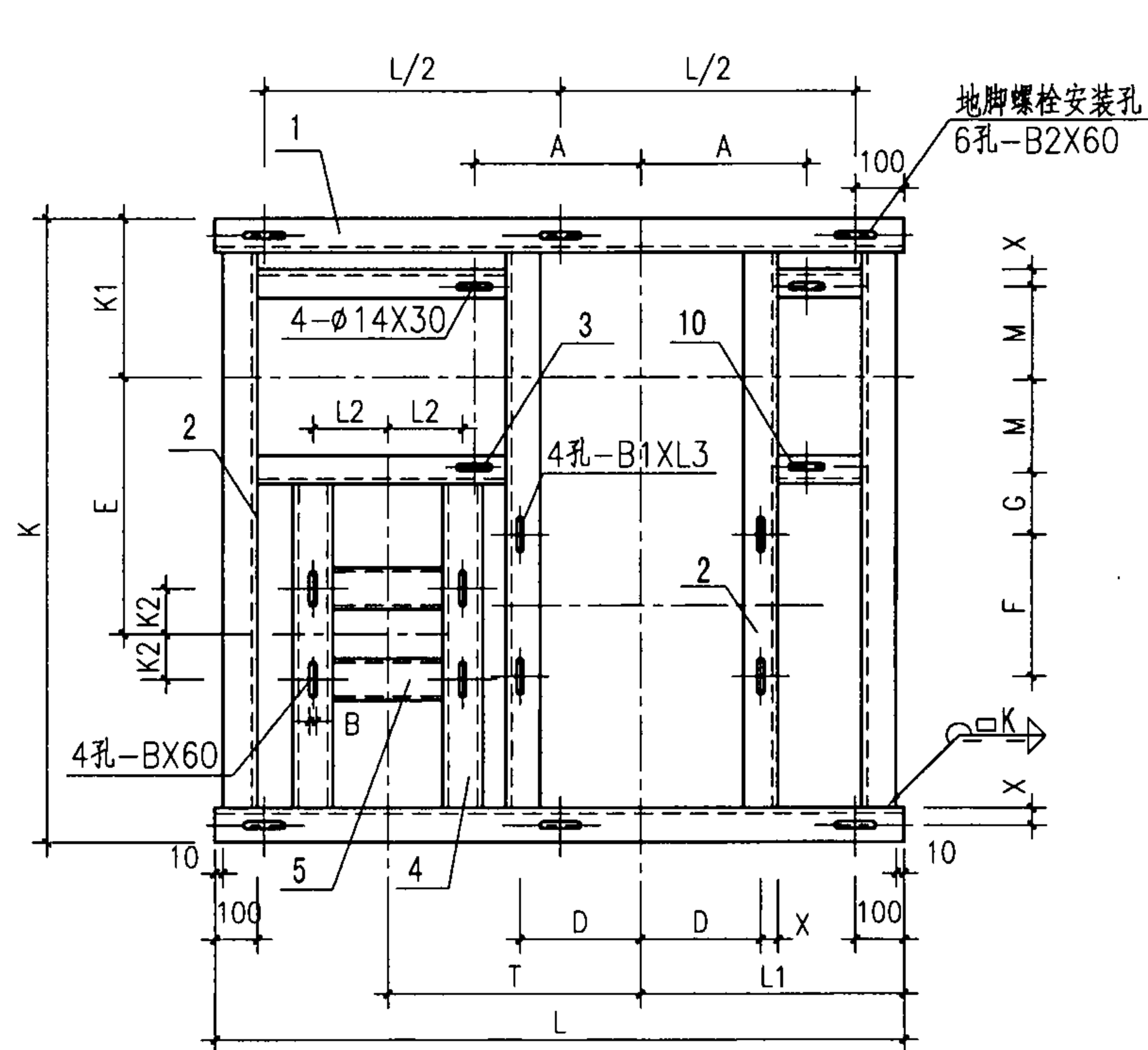
底架详图
