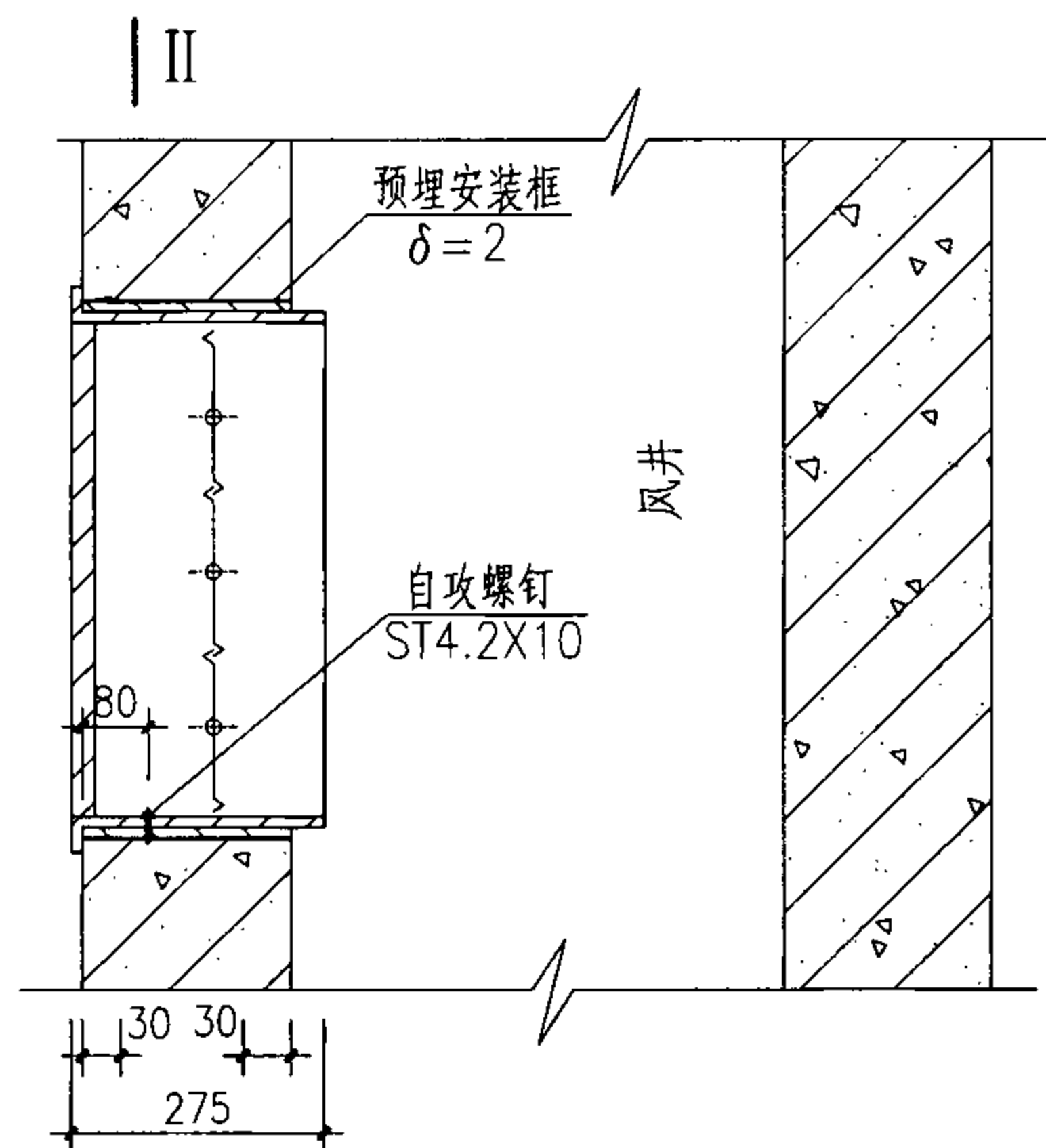
I-I (混凝土墙上安装)
