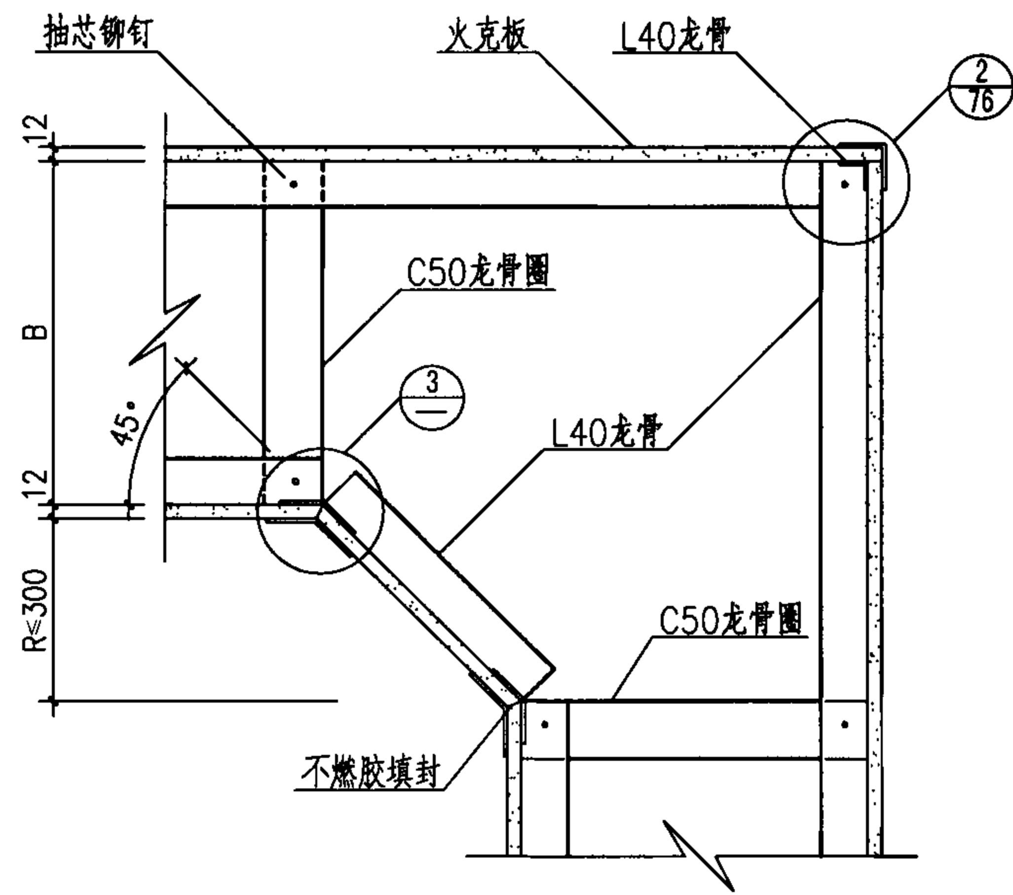
防火风管弯头 (R≤300mm)
