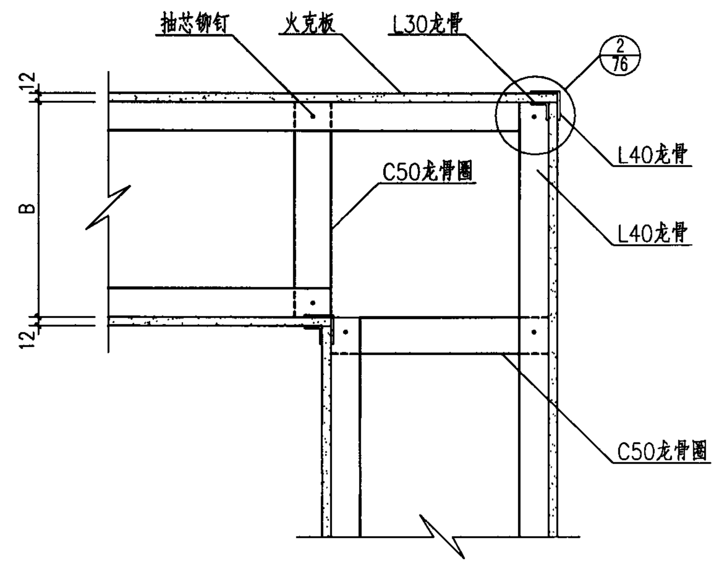
防火风管弯头 (R≤300mm)
