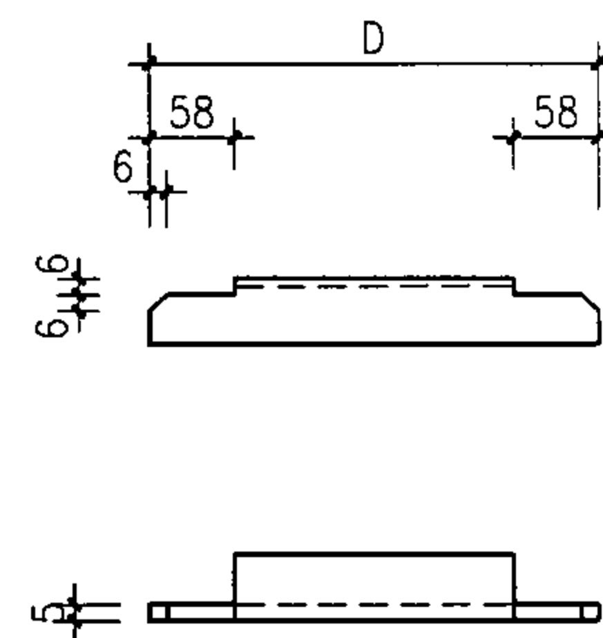
件号4详图
