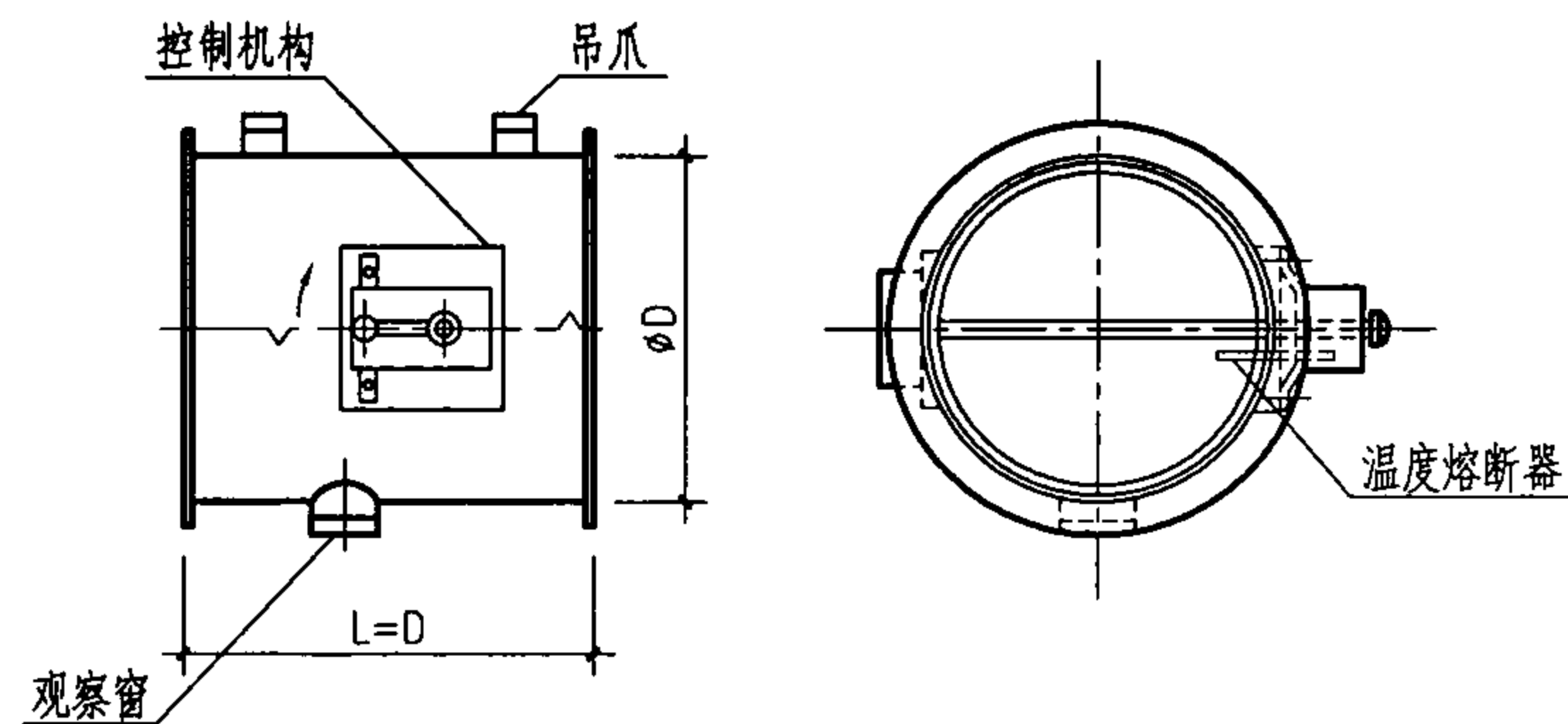
圆形防火阀
