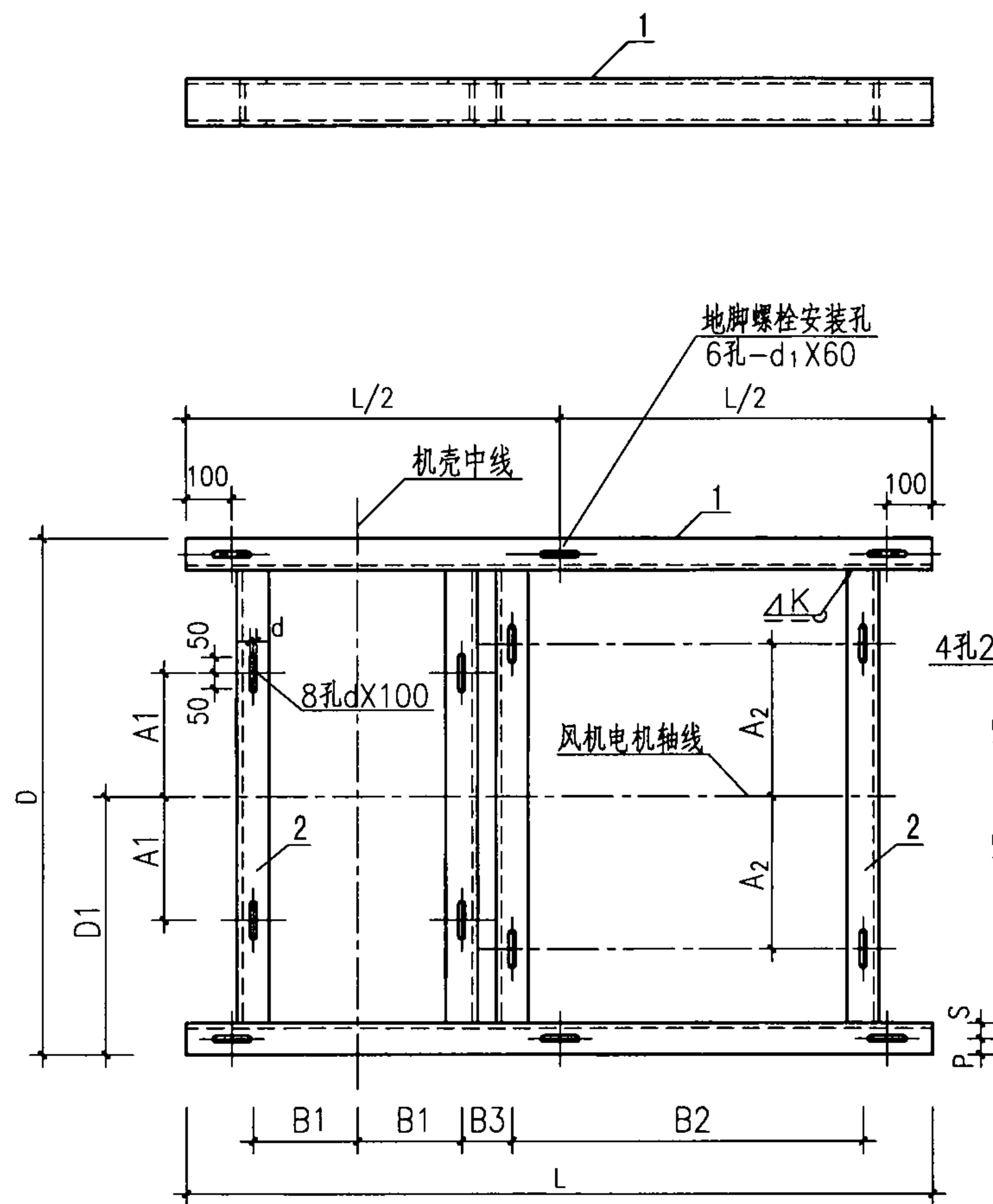
底架详图
