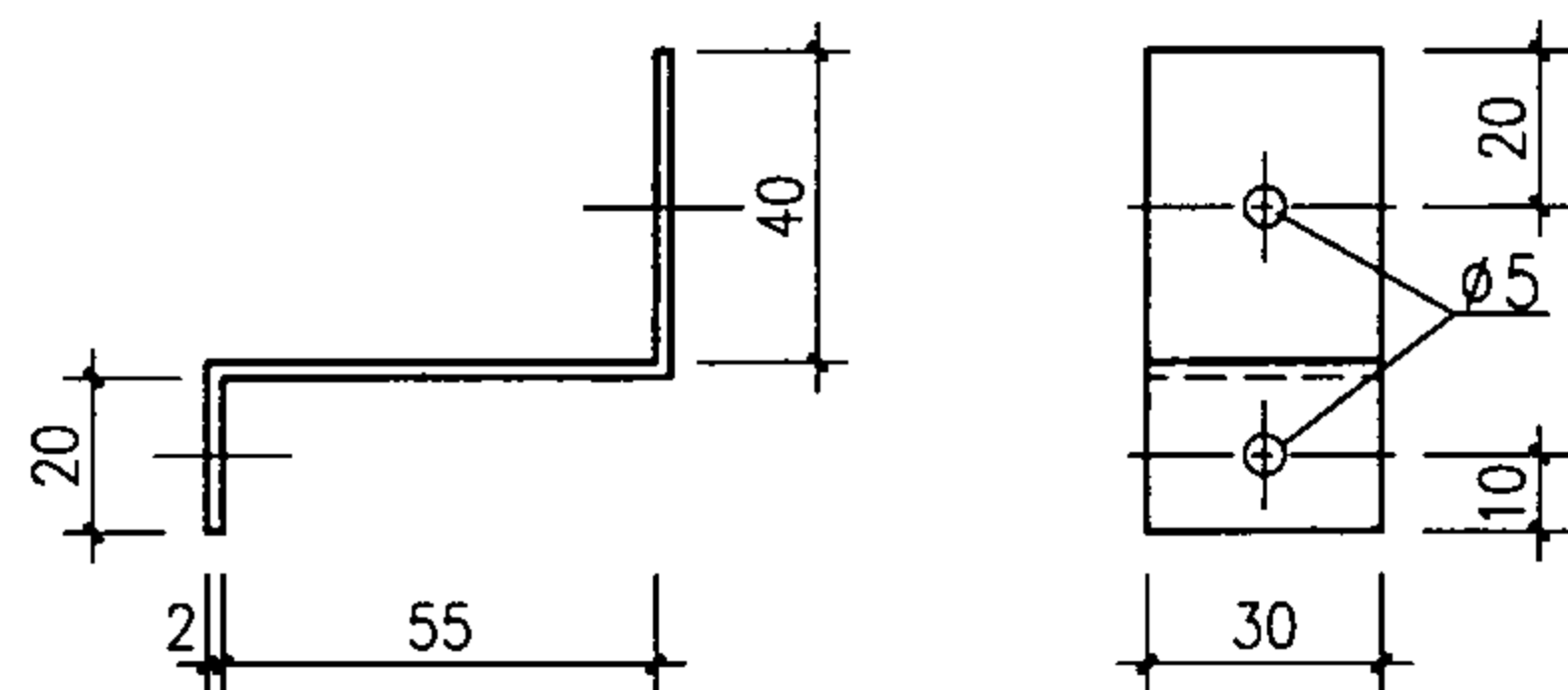
扁钢卡件
