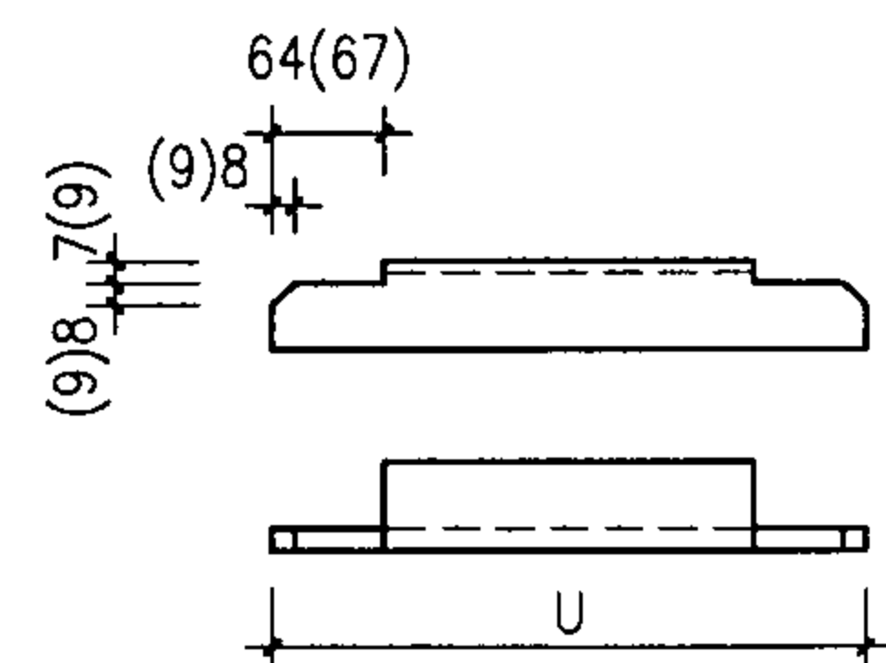
件号7详图
