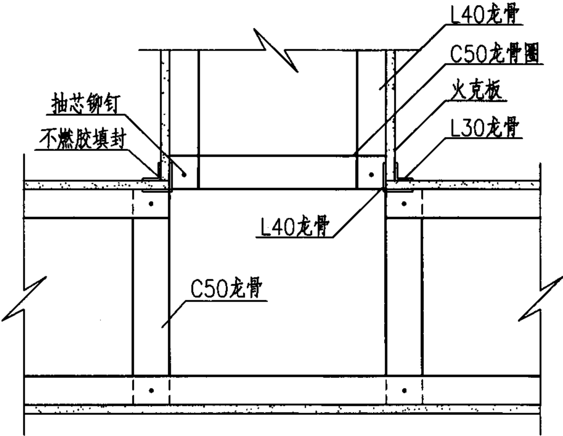
防火风管三通、变径及大样图
