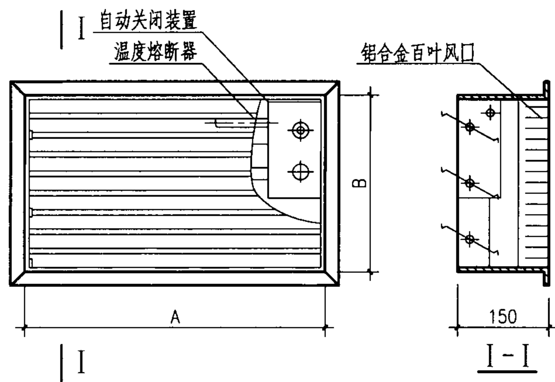
防火风口
